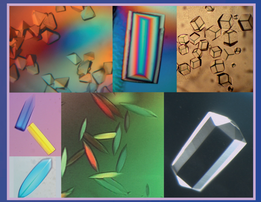
Différents cristaux biologiques «cultivés» pour la détermination de leur structure. © IUCr journals
