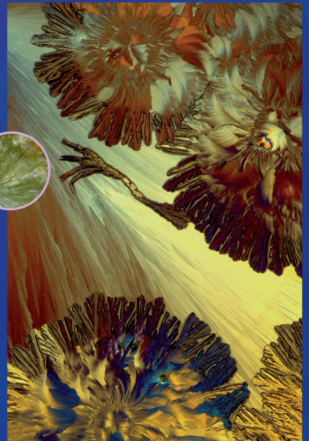
Recristallisation d'acide citrique, Jeanne Michaud IMPMC - Paris. © CNRS-Images
