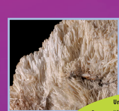
Cerussite
